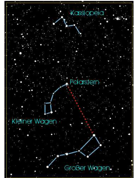
Der nördliche Abendhimmel. Anstatt „Wagen“ sagt man auch „Bär“.
